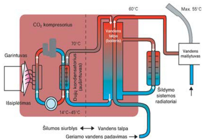
„SANYO CO 2 ECO šilumos siurblio ir namo šildymo sistemos veikimo schema“
